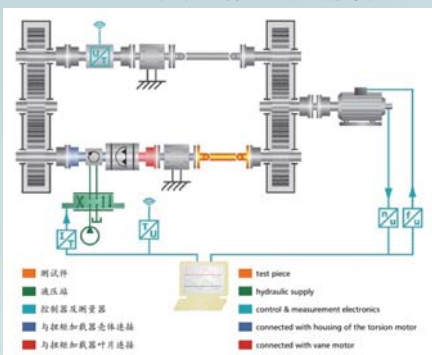
扭矩加载实验台结构示意图
