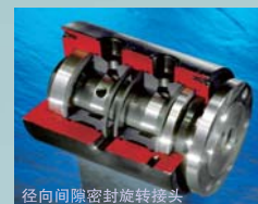
径向间隙密封旋转接头
